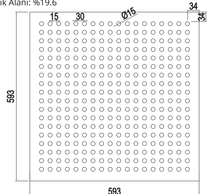
15mm YUVARLAK Delik Alanı: %19.6
